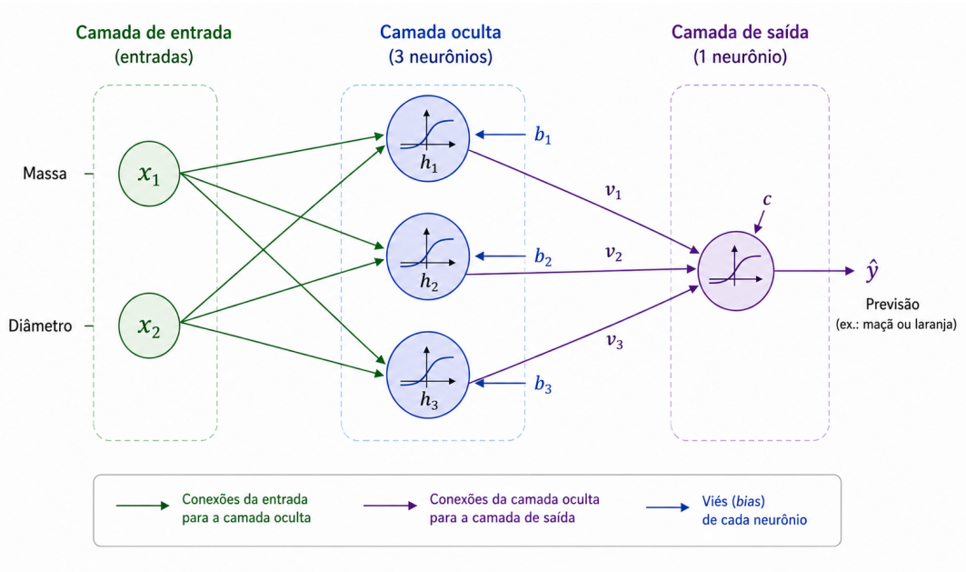
Figura 5: Arquitetura pedagógica 2–3–1 usada para introduzir o funcionamento de uma rede neural. As duas entradas — massa e diâmetro — alimentam três neurônios na camada oculta, cujas ativações h_1 , h_2 , h_3 são combinadas por um neurônio de saída para produzir a previsão \hat{y} . Cada conexão possui um peso ajustável, e cada neurônio possui um viés associado.
